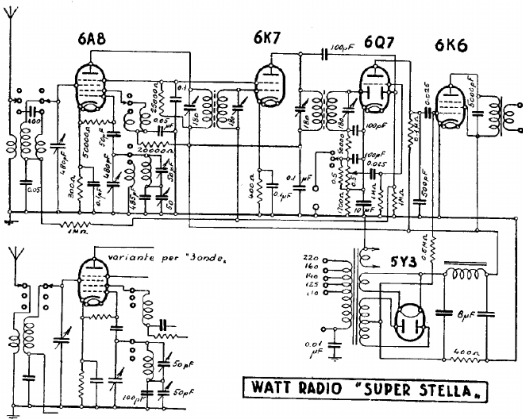
WATT RADIO. — Mod. « Super Stella » e « Super Stella Fono ». — Produzione 1940-1941. Media frequenza: 460 kHz.
